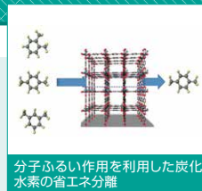
分子ふるい作用を利用した炭化水素の省エネ分離
